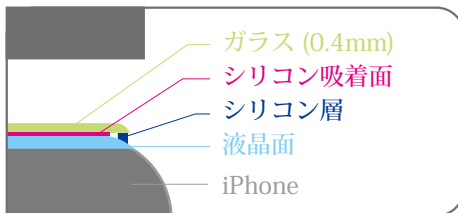
断面図
