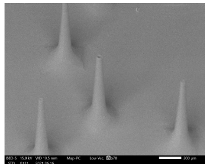
医療用中空型マイクロニードルのSEM像
